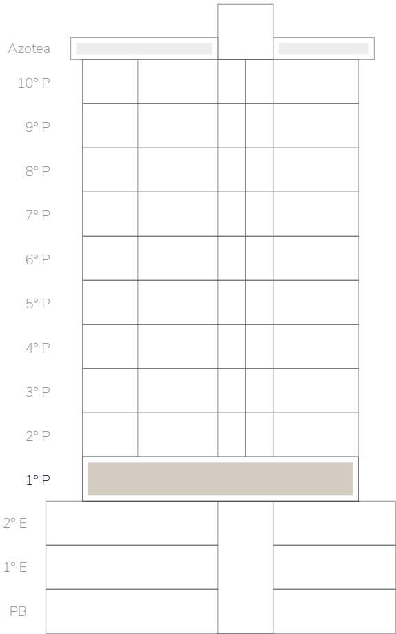
CORTE ESQUEMÁTICO
