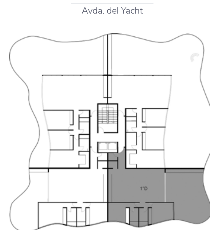
UBICACIÓN EN PLANTA
